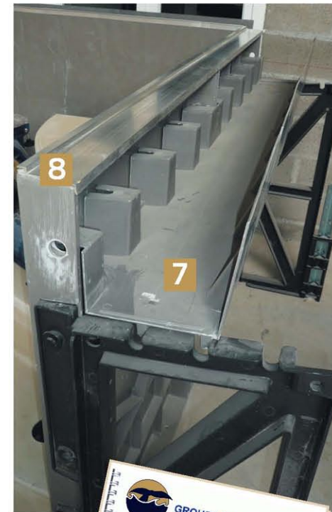
Bassin bloc à bancher de 28 x 4 m à débordement
